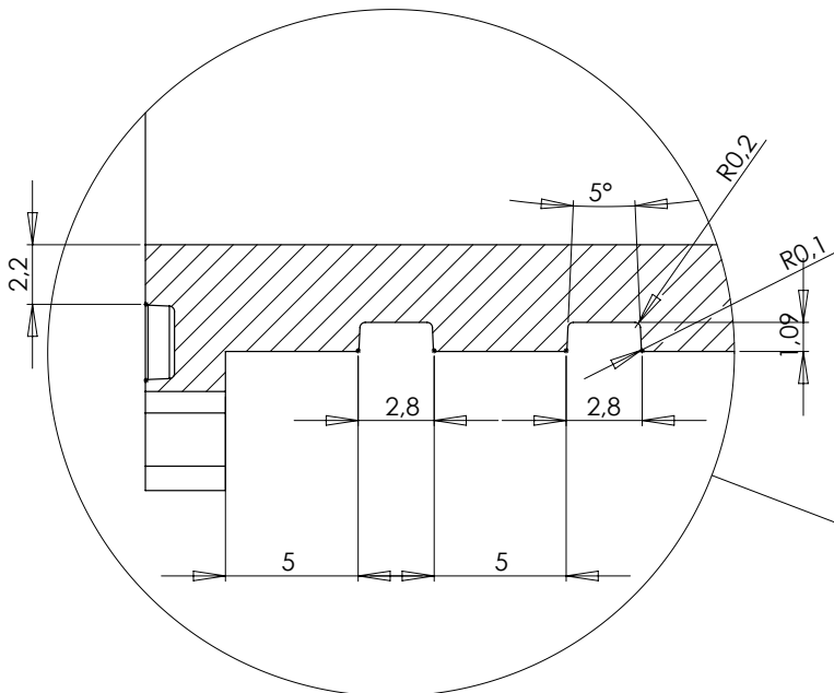
DÉTAIL B
