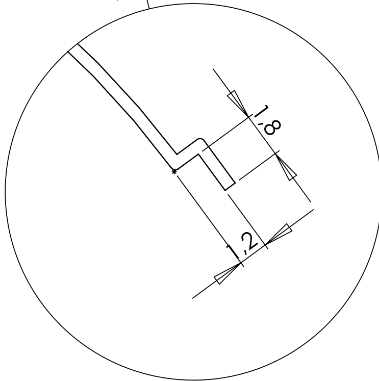
DÉTAIL A
