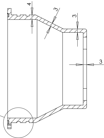
COUPE A-A
