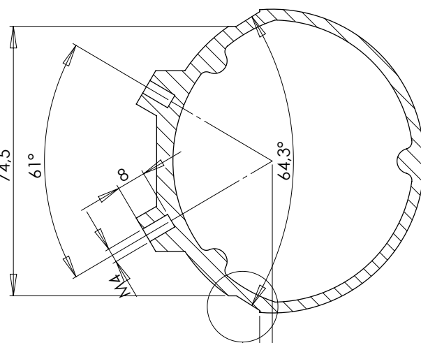
COUPE A-A
