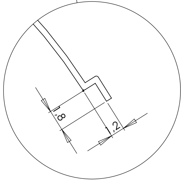
DÉTAIL A
