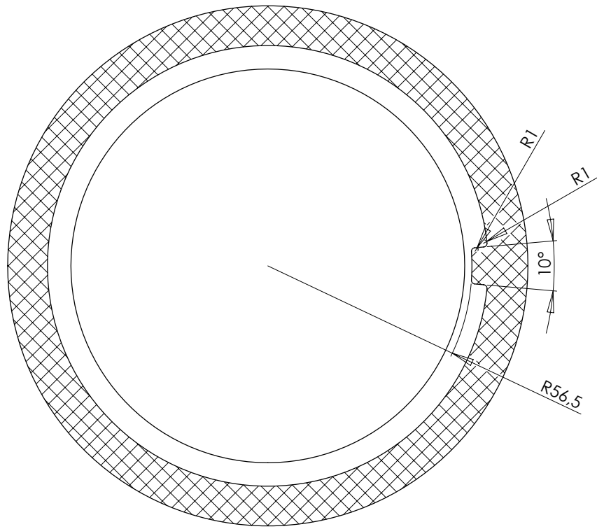
COUPE B-B
