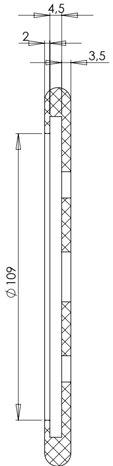
COUPE A-A
