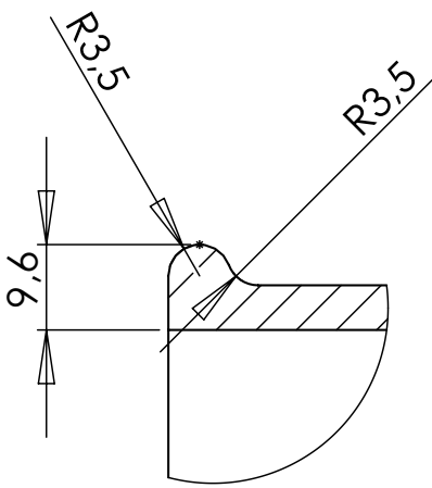
DÉTAIL B
