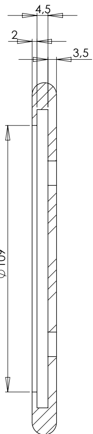
COUPE A-A
