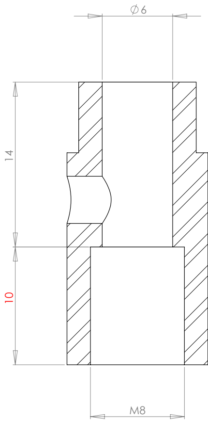
COUPE A-A
