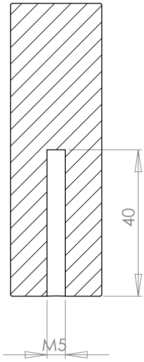
COUPE A-A
