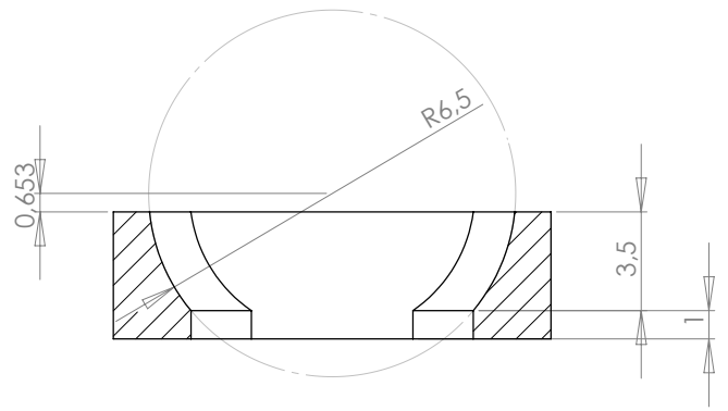
COUPE A-A
