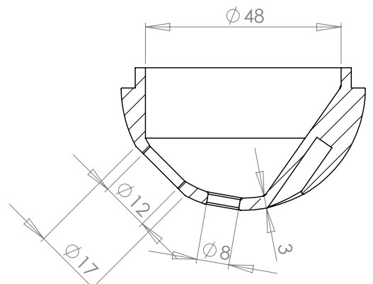
COUPE A-A
