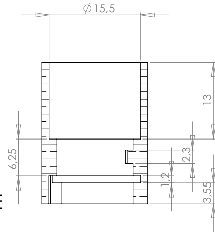
COUPE A-A
