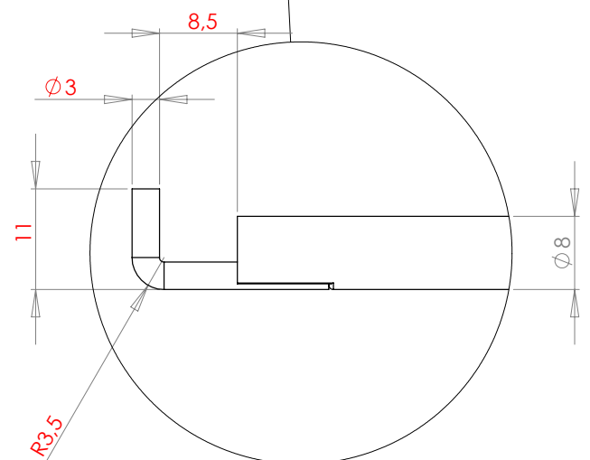
DÉTAIL A
