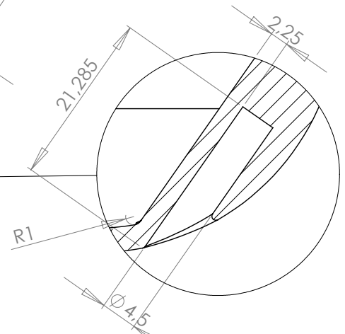
DÉTAIL C
