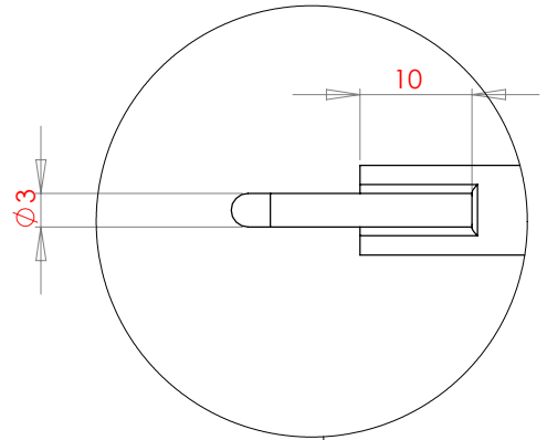
DÉTAIL C
