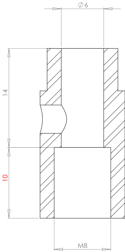
COUPE A-A
