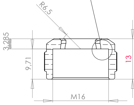
COUPE A-A
