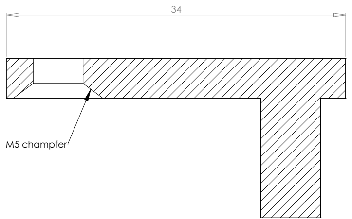
COUPE A-A
