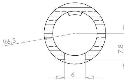
COUPE E-E
