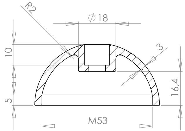
COUPE A-A
