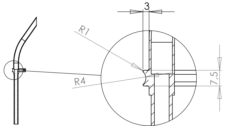
DÉTAIL D
