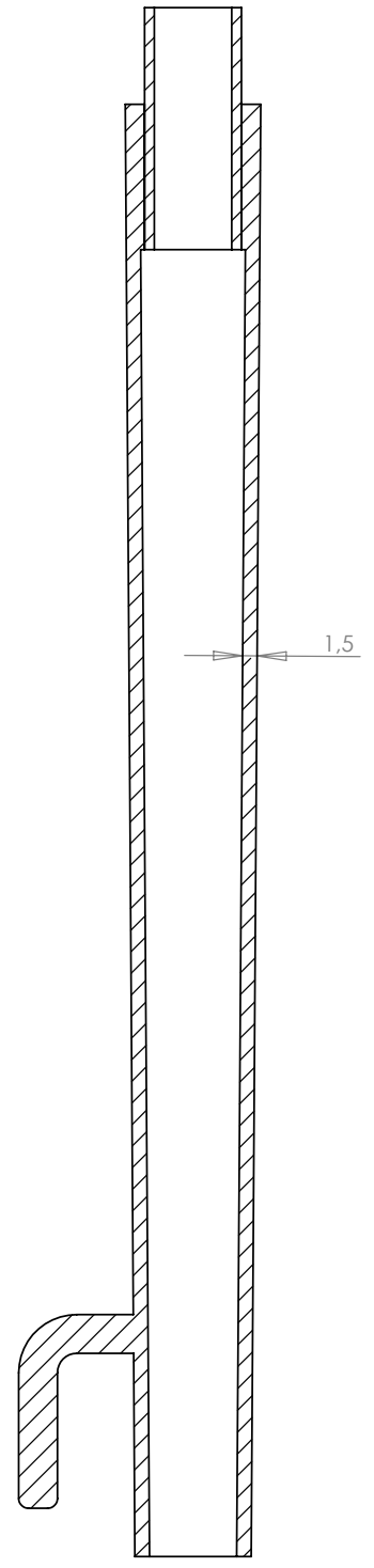
COUPE A-A
