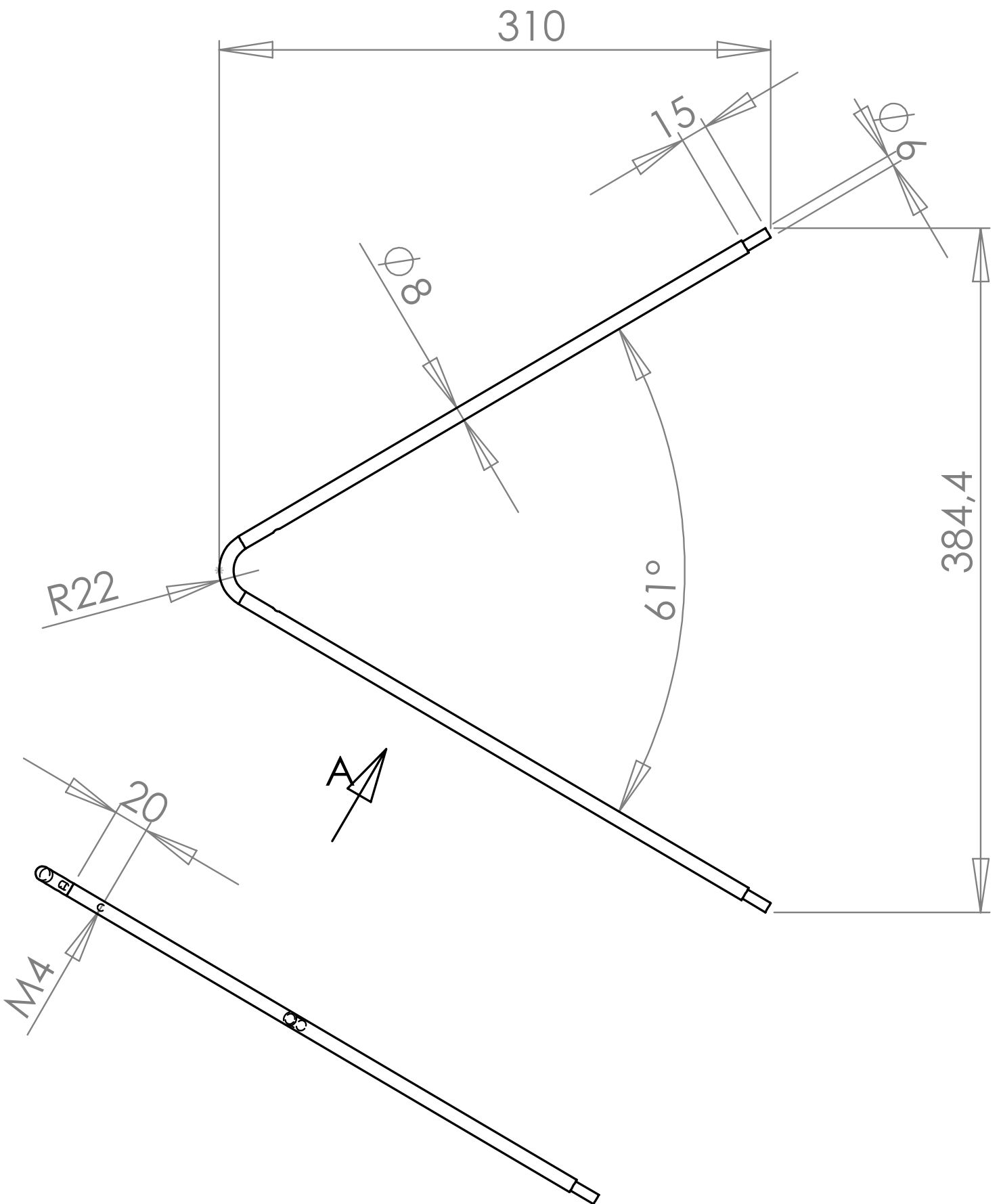
VUE A
