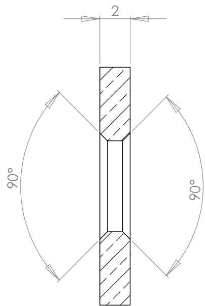
COUPE A-A
