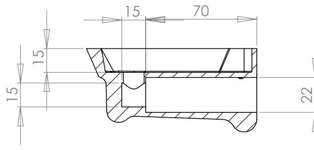
COUPE A-A
