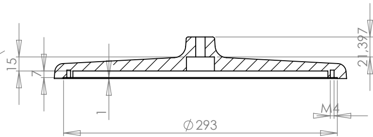
COUPE A-A
