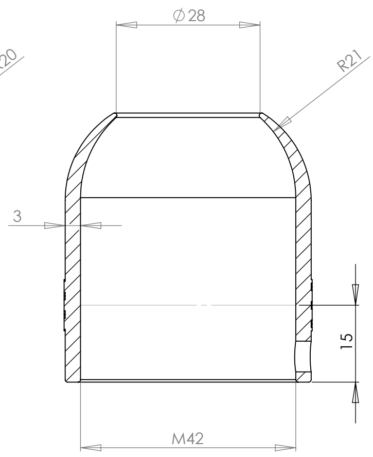
COUPE A-A
