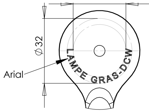
DÉTAIL B
