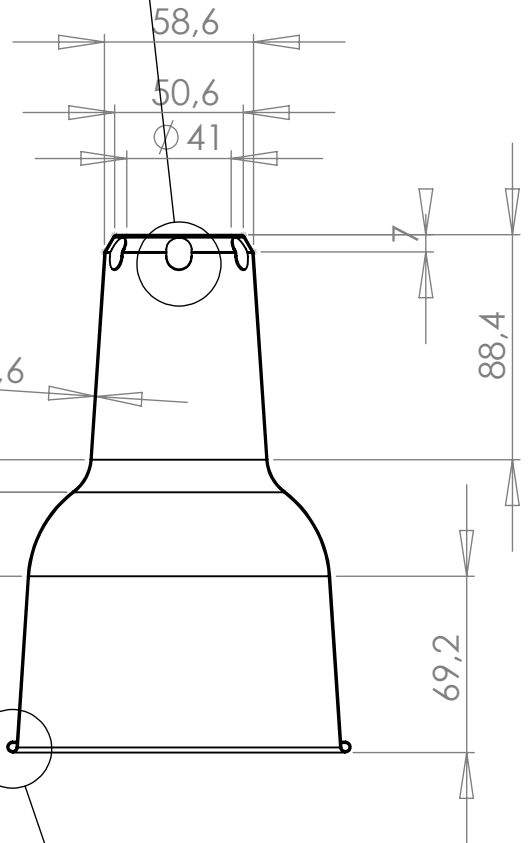
COUPE A-A
