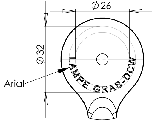
DÉTAIL B
