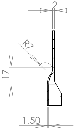
COUPE C-C
