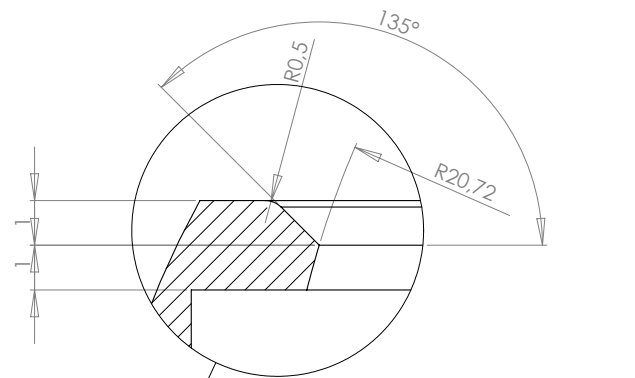
DÉTAIL B
