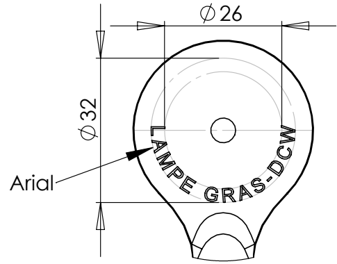
DÉTAIL B
